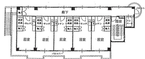
2階・3階平面図
