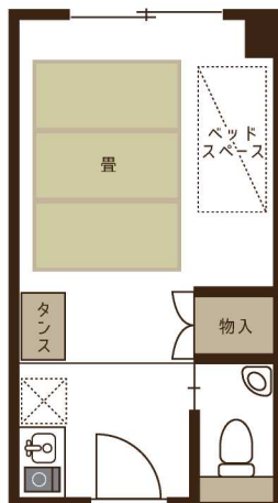
居室詳細図
